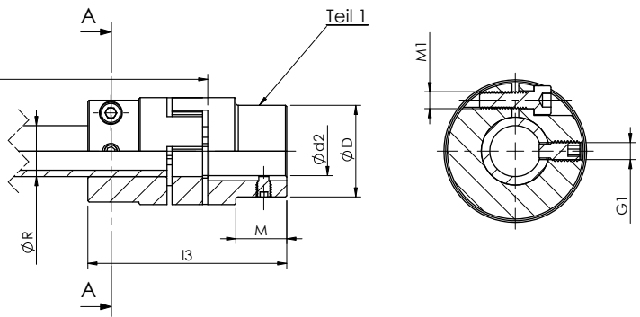
SNITT A-A
